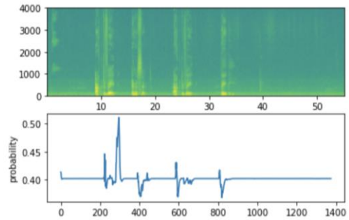
(그림 6) Keyword Spotting 모델 적용 결과
